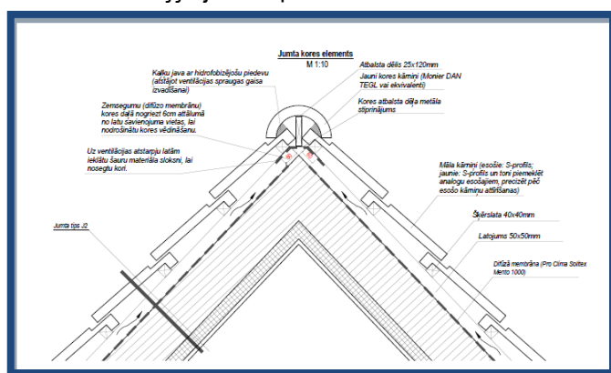
29. att. Vēdināmais jumts. Esošās konstrukcijas un pievienojamie materiāli, to raksturojums, lai izveidotu siltinātu vēdināmo jumtu. Rasējums no projekta. 21
